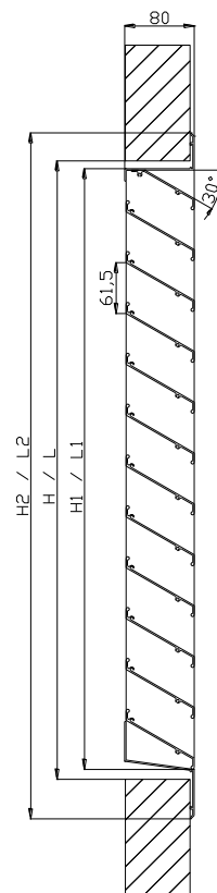
FA-450 – ΤΟΜΗ
