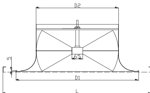
SW-1400-P – ΤΟΜΗ
