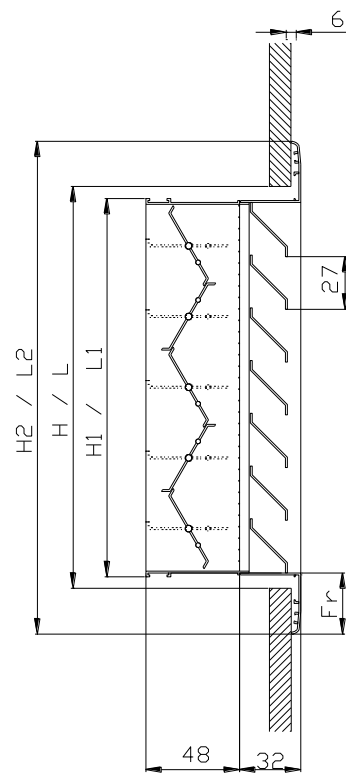
FA-400-D – ΤΟΜΗ ΜΕ DAMPER
