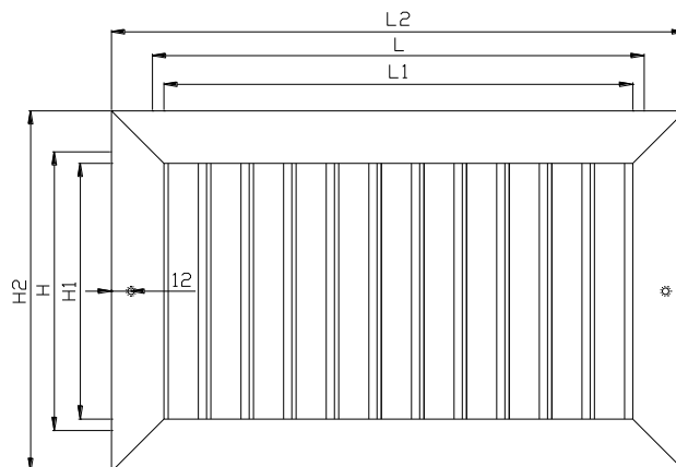
FA-400 – ΟΨΗ (H x L)
