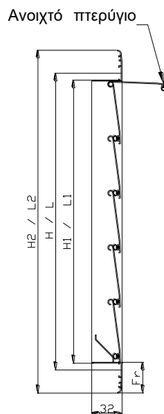
NR-900 - ΤΟΜΗ
