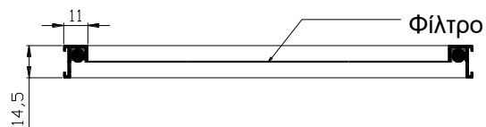
ΦΙΛΤΡΟ – ΤΟΜΗ
