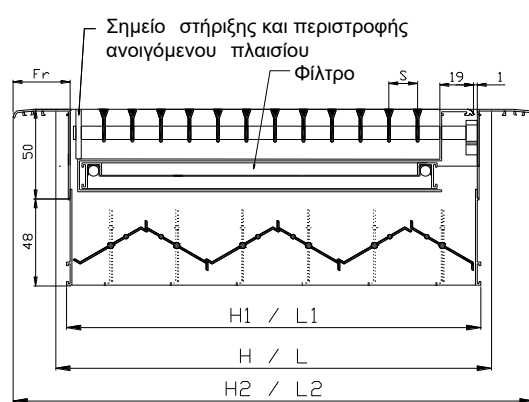
LF-201-D-A-F – ΤΟΜΗ ΜΕ DAMPER
