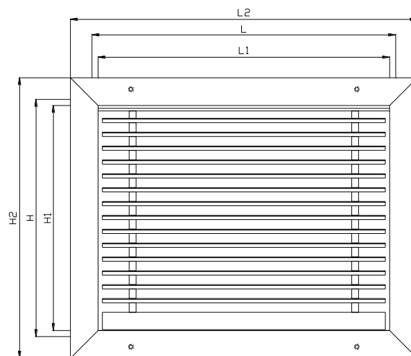
LF-202-A – ΟΨΗ
