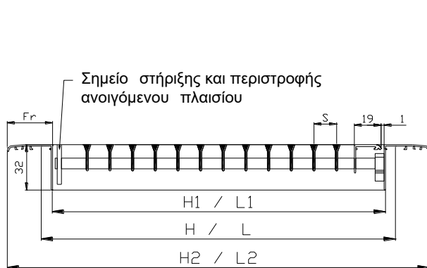
LF-201-A – ΤΟΜΗ
