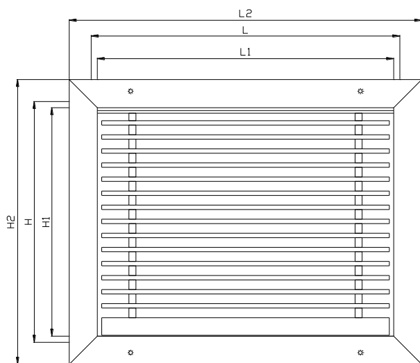
LF-201-A – ΟΨΗ
