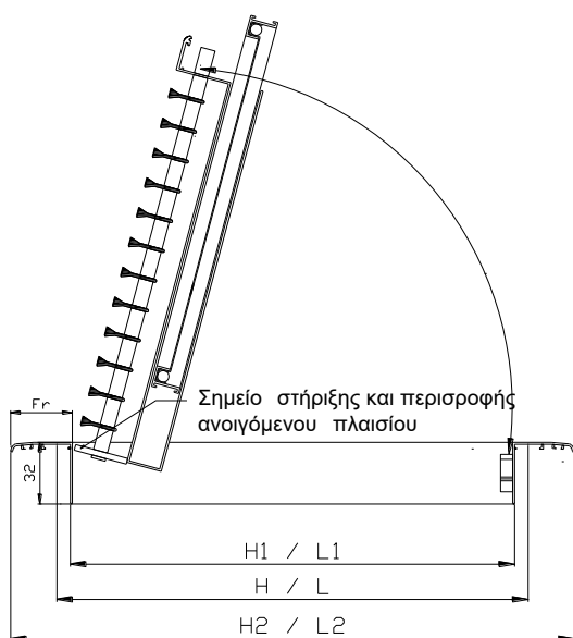
LF-201-A-F – ΤΟΜΗ
