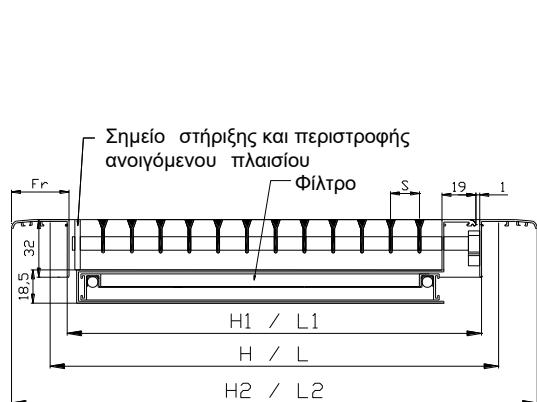
LF-201-A-F – ΤΟΜΗ
