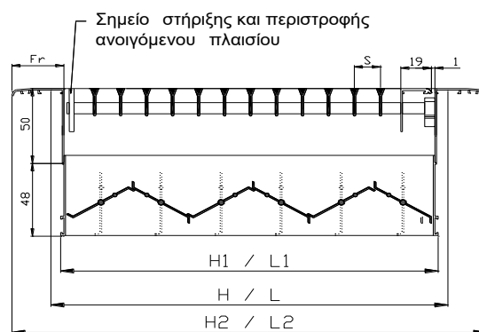
LF-201-D-A – ΤΟΜΗ ΜΕ DAMPER
