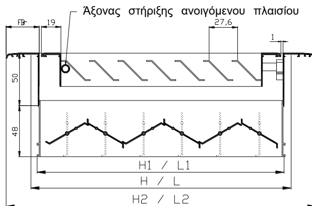
FA-400-D-A – ΤΟΜΗ ΜΕ DAMPER
