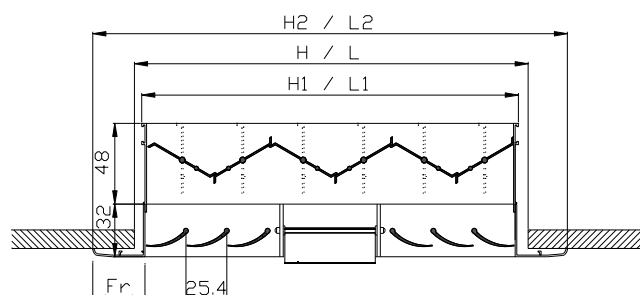
CM-503-D – ΤΟΜΗ ΜΕ DAMPER
