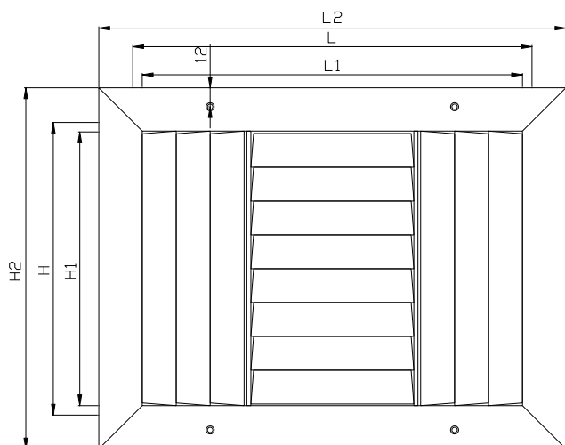
CM-503 – ΟΨΗ (L x H)
