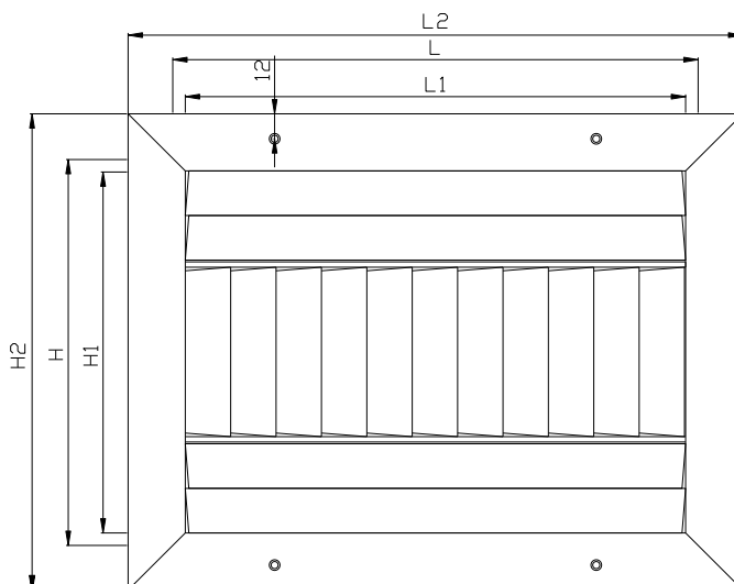
CM-503 – ΟΨΗ (H x L)
