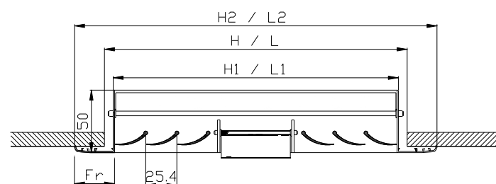
CM-503-E – ΤΟΜΗ ΜΕ ΕΣΧΑΡΑ
