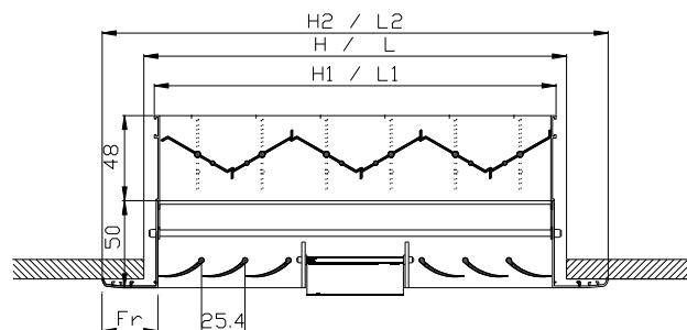
CM-503—D-E – ΤΟΜΗ DAPER ΚΑΙ ΕΣΧΑΡΑ
