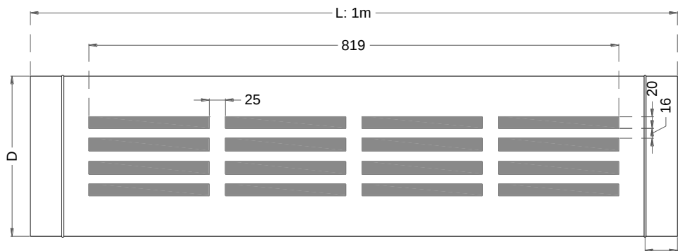
SW-TUBE – ΟΨΗ
