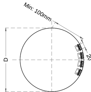
SW-TUBE – ΤΟΜΗ
