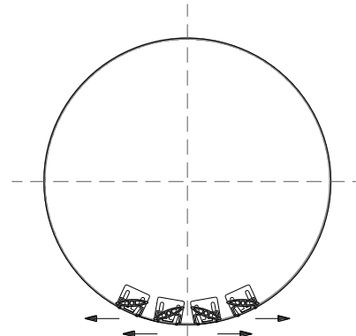
SW-TUBE – ΤΟΜΗ – ΟΡΙΖΟΝΤΙΑ ΡΟΗ 2 ΚΑΤΕΥΘΥΝΣΕΩΝ
