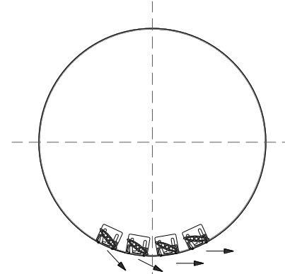
SW-TUBE – ΤΟΜΗ – ΟΡΙΖΟΝΤΙΑ ΡΟΗ 1 ας ΚΑΤΕΥΘΥΝΣΗΣ
