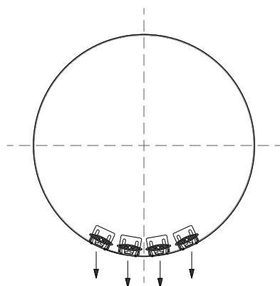
SW-TUBE – ΤΟΜΗ – ΚΑΘΕΤΗ ΡΟΗ
