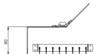
DAMPER ΤΥΠΟΥ ΠΕΤΑΛΟΥΔΑΣ ΜΕ ΕΣΧΑΡΑ - ΤΟΜΗ
