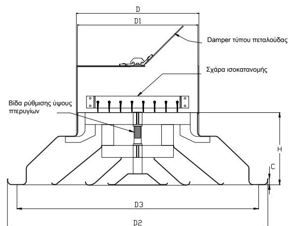
CR-700-D-E – ΤΟΜΗ ΜΕ ΕΣΧΑΡΑ ΚΑΙ DAMPER
