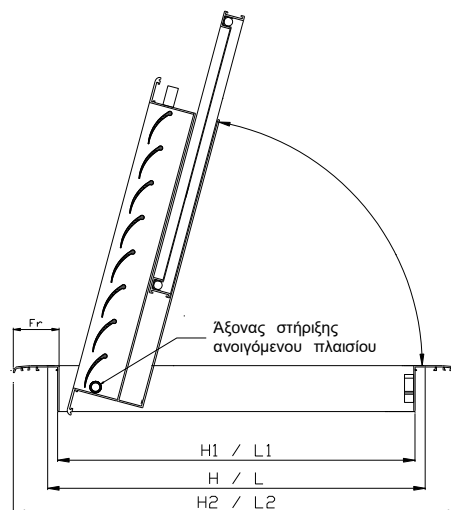
CM-501-A-F - ΤΟΜΗ
