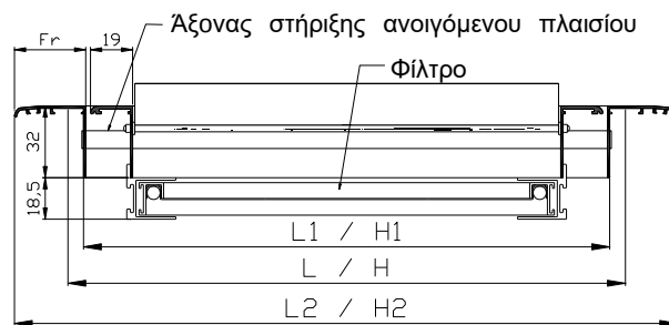
CM-501-A-F - TOMEΣ
