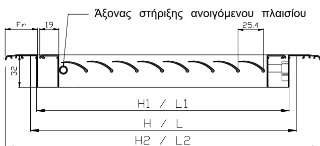
CM-501-A – ΤΟΜΕΣ
