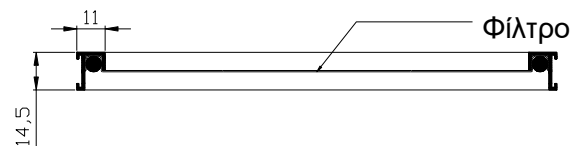
ΦΙΛΤΡΟ - ΤΟΜΗ
