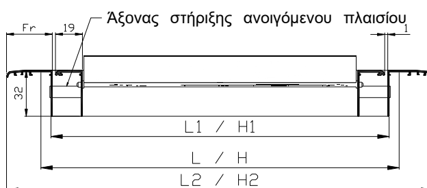
CM-501-A – ΤΟΜΕΣ
