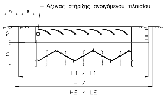
CM-501-D-A – ΤΟΜΗ ΜΕ DAMPER
