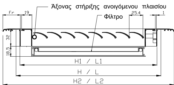
CM-501-A-F - TOMEΣ
