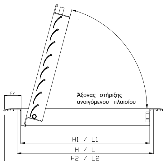
CM-501-A – ΤΟΜΗ
