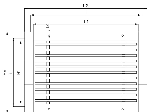
TL-201/211 – ΟΨΗ
