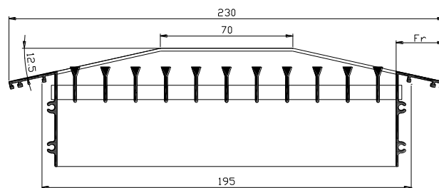
TL-201/211 – TOMH (L x 195 mm)
