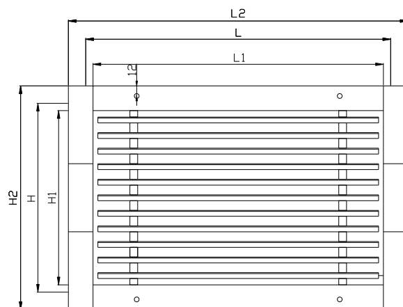
TL-202/212 – ΟΨΗ
