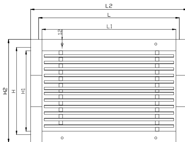
TL-202-2/212-2 – ΟΨΗ
