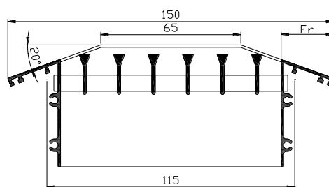
TL-201/211 – ΤΟΜΗ (L x 115 mm)
