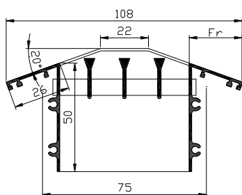
TL-201/211 – ΤΟΜΗ (L x 75 mm)
