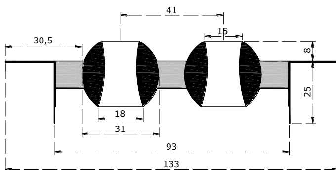
Φ15 MULTIJET 2 – ΤΟΜΗ
