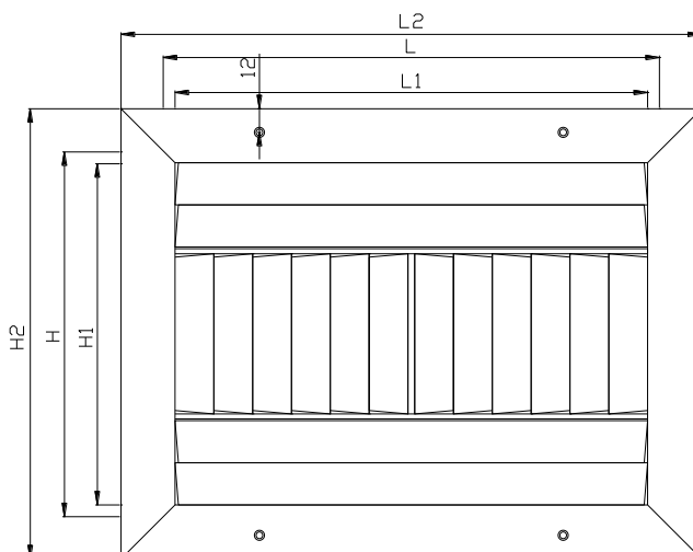
CM-504 – ΟΨΗ (H x L)
