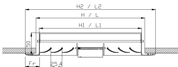
CM-504-E – TOMH ME ΕΣΧΑΡΑ
