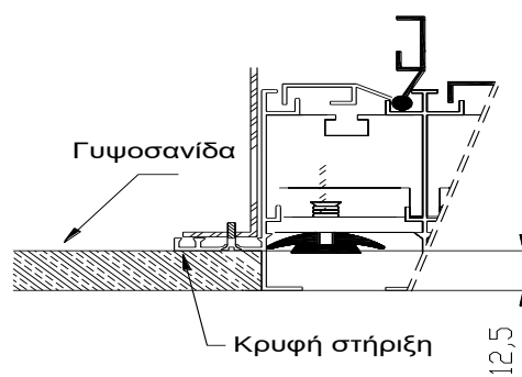
SL-850 – ΛΕΠΤΟΜΕΡΕΙΑ ΤΟΠΟΘΕΤΗΣΗΣ
