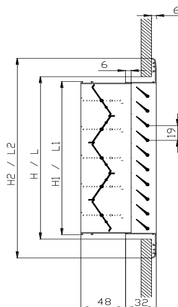
WR-150-D – TOMH ME DAMPER
